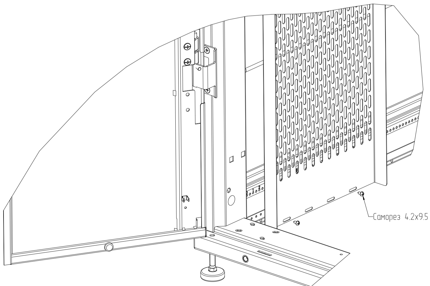
Установка ВКО в шкафы серии D9000
