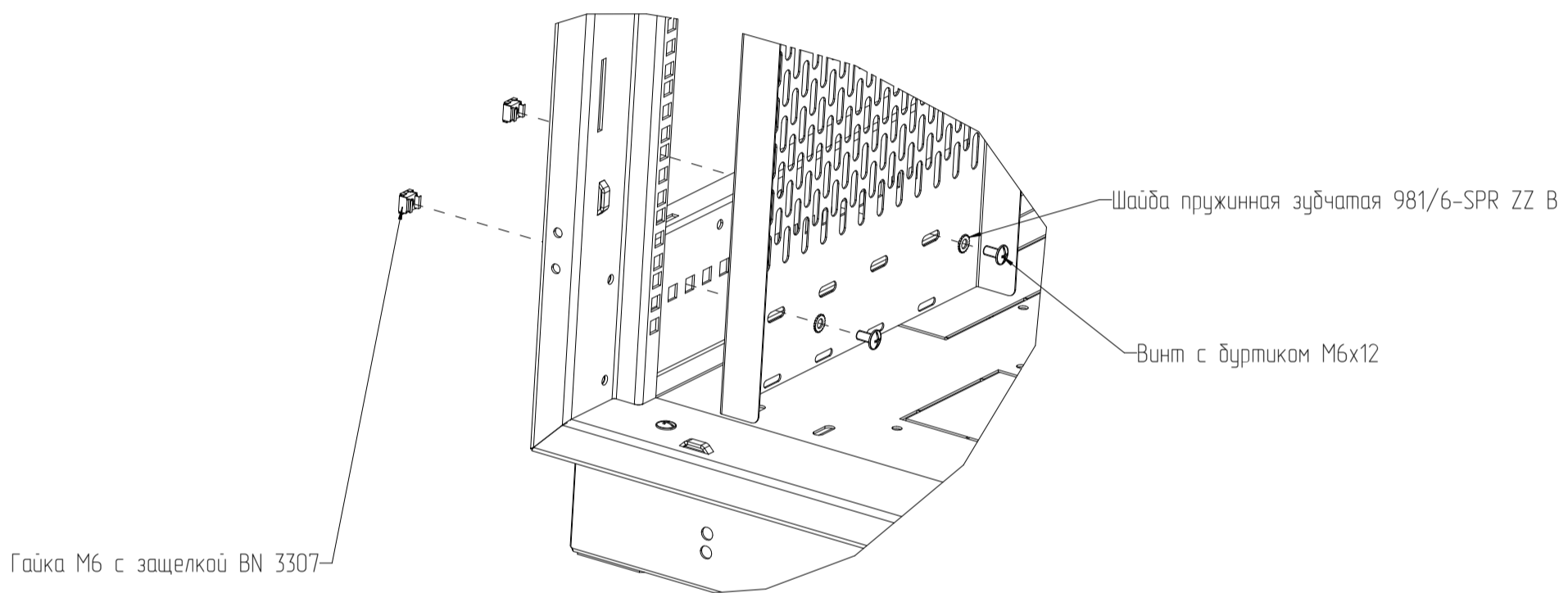
Установка ВКО в шкафы серии S3000
