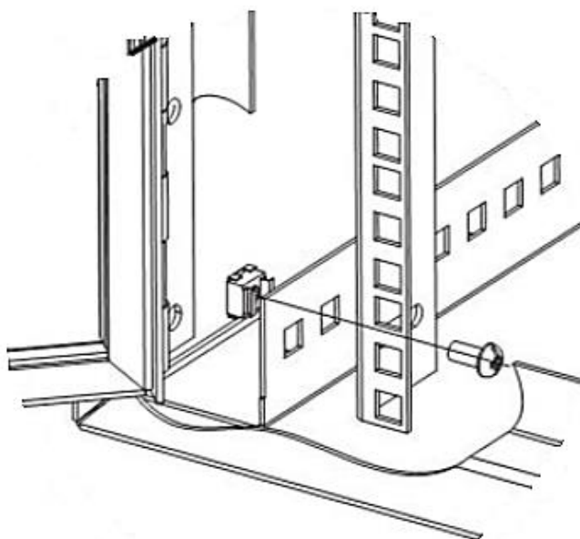
Рисунок 1. Установка 19" направляющих в шкаф D9000
