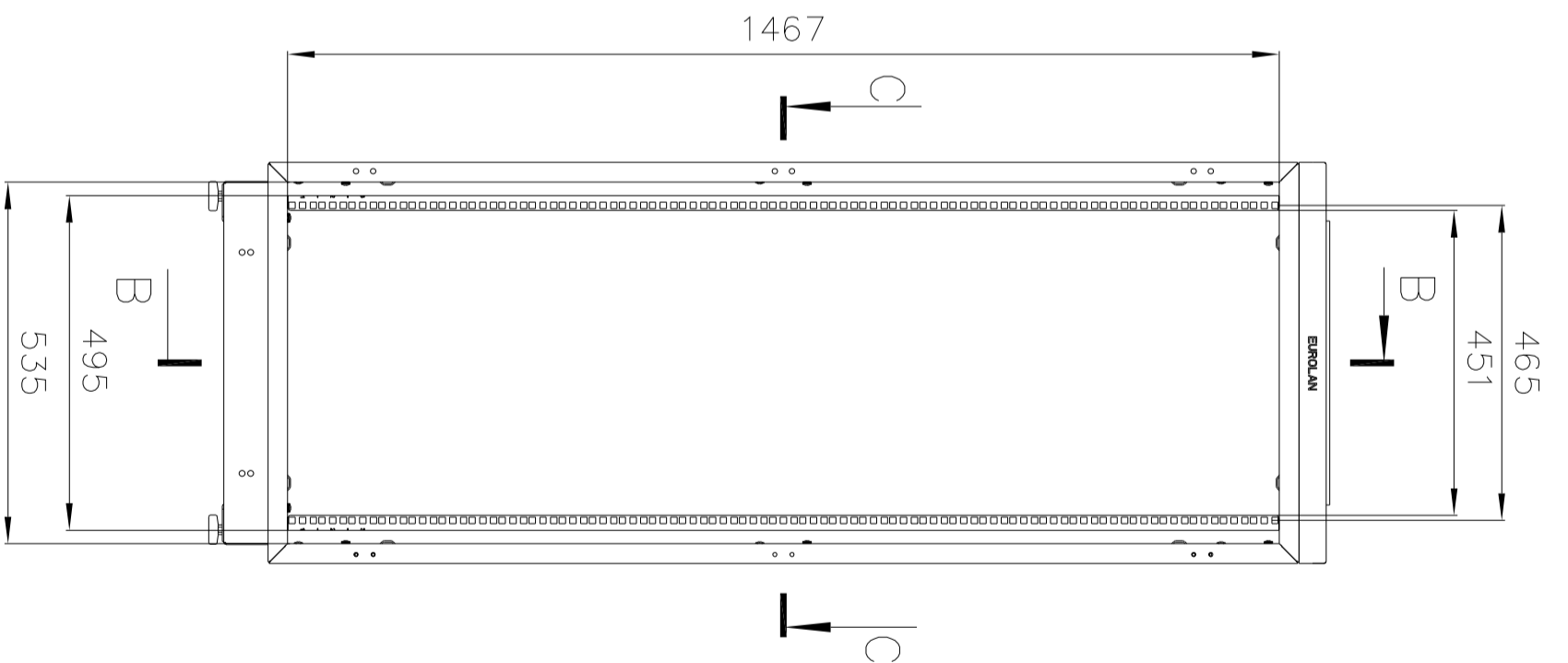
Вид каркаса
