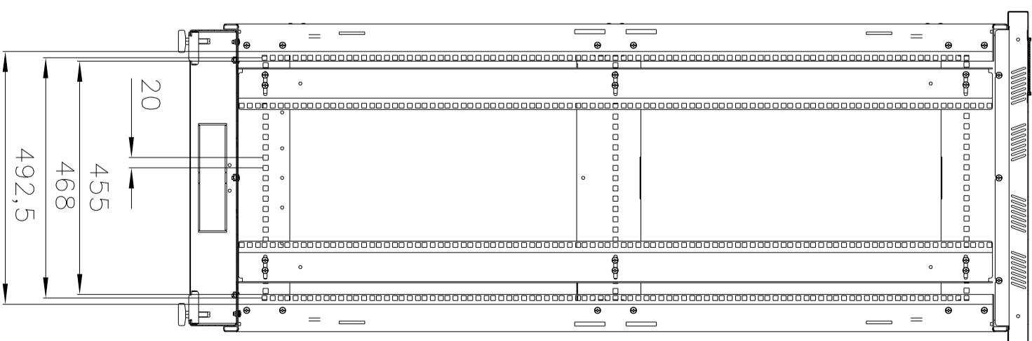
B-B
