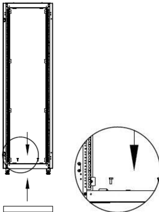
Рисунок 1. Установка крепления к раме шкафа.
